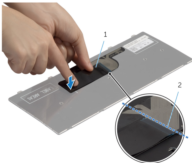
1 键盘电缆
